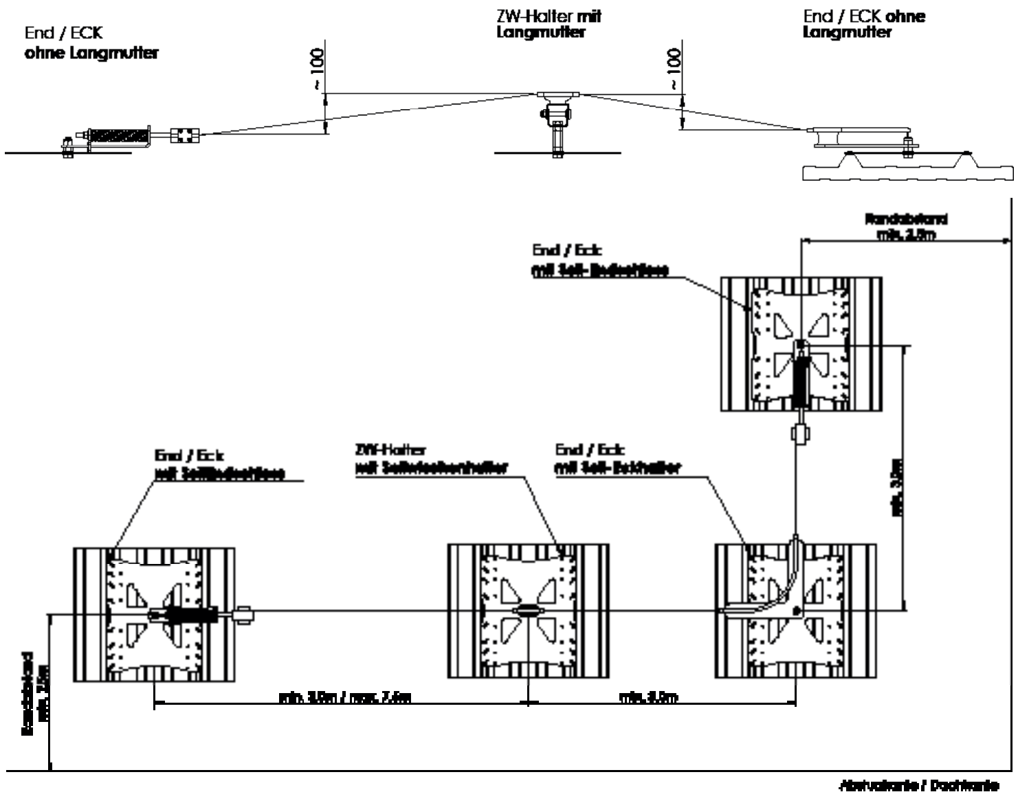
Skizze "Sturzfaktor"
